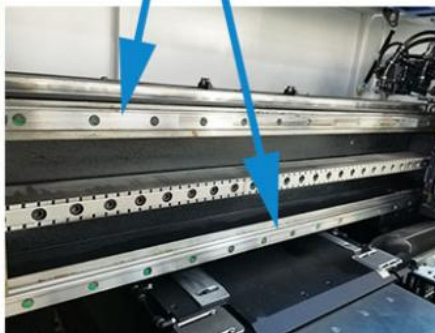
Linear motor
